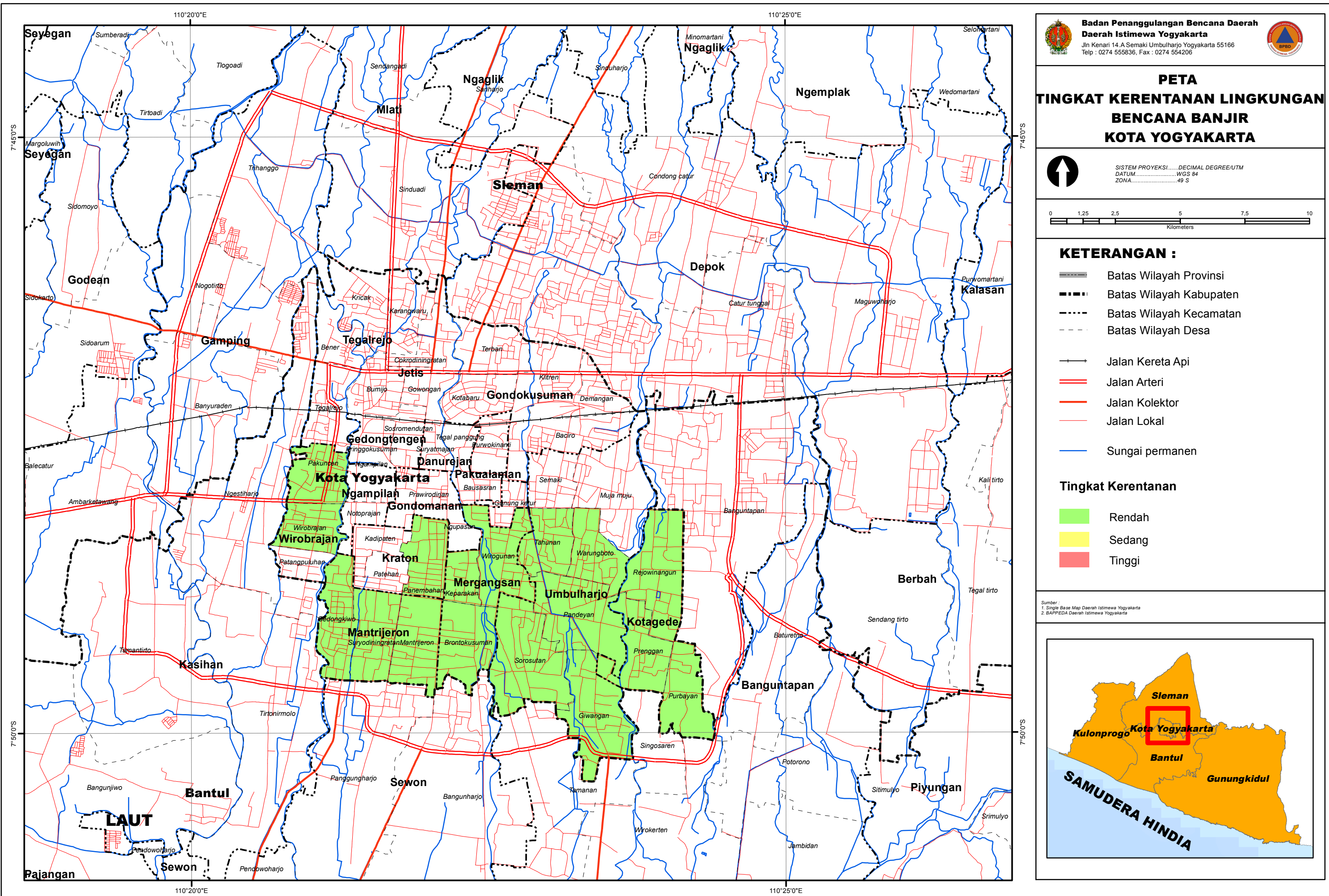
Gambar 5.20. Peta Tingkat Kerentanan Lingkungan Bencana Banjir Kota Yogyakarta
